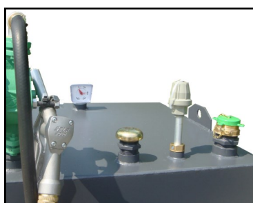
Detail tankset 3C gemonteerd op tank
